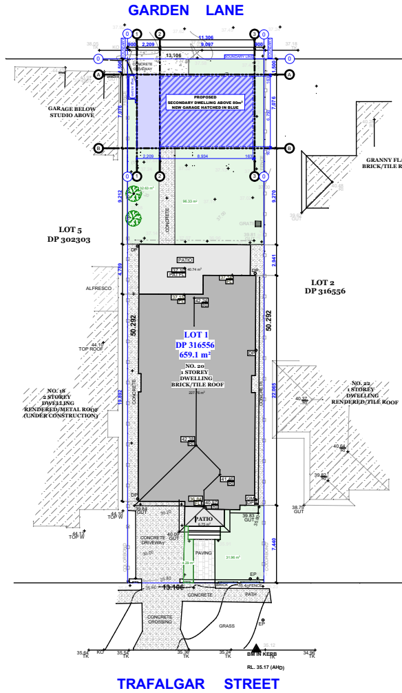
1 SITE PLAN 1:500
